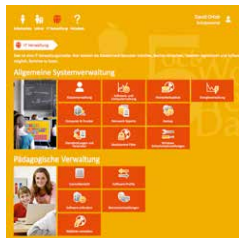
SkoolControl-Benutzeroberfläche.
